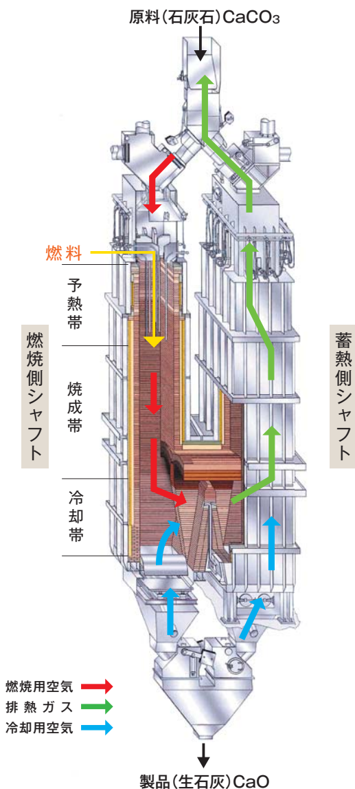
Maerz® 型焼成炉(並行流蓄熱式)
