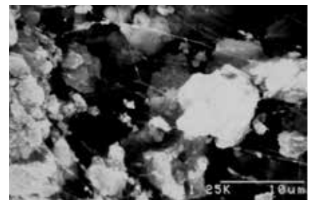
スーパーアースライムの顕微鏡写真 サブミクロン径のPTFE繊維が安定材粒子を捕らえ発塵を防止します。
